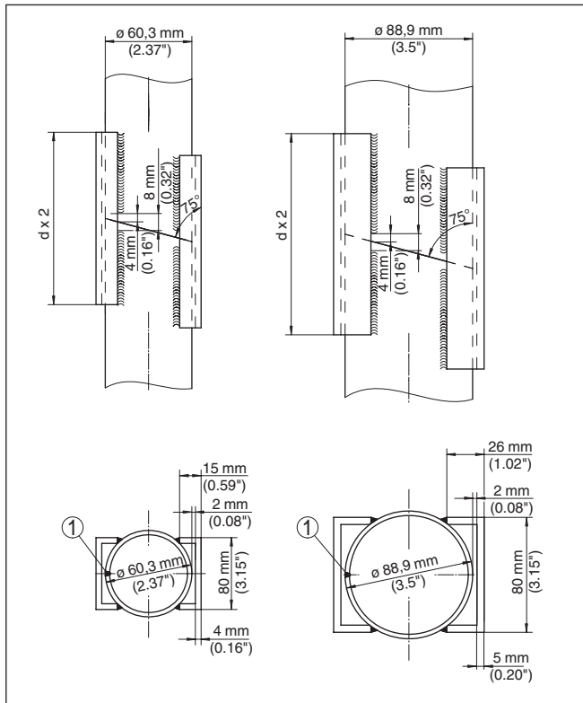
Fig. 12: Soudure sur prolongation de tube tranquillisateur pour différents exemples de diamètres
