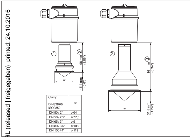
Abbildung 40: LEVEL TRANSMITTER 8138, Hygieneanschluss 2
