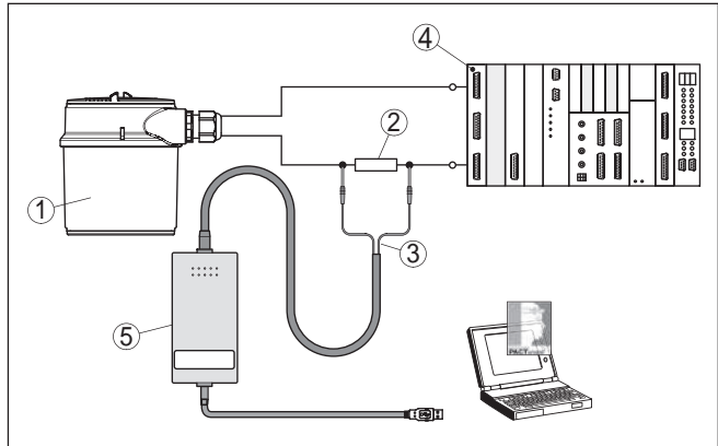
Abb. 19: Anschluss des PCs via HART an die Signalleitung
