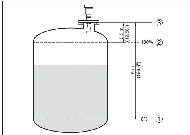
Fig. 18: Parameter adjustment example min./max. adjustment
