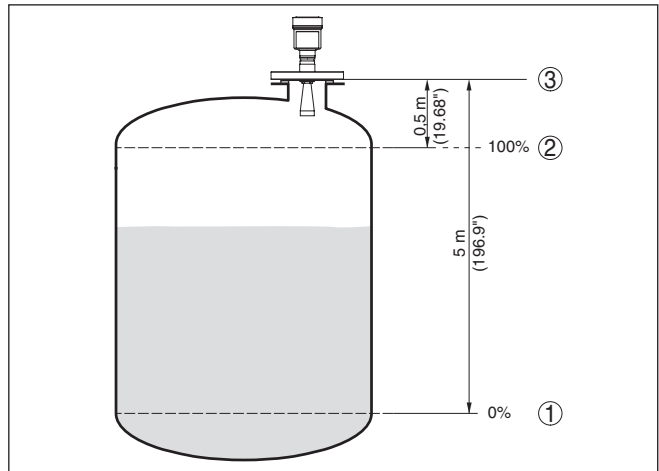
Fig. 18: Exemple de paramétrage réglage min./max.
