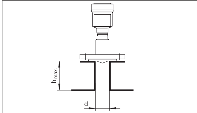
Abb. 7: Abweichende Rohrstutzenmaße
