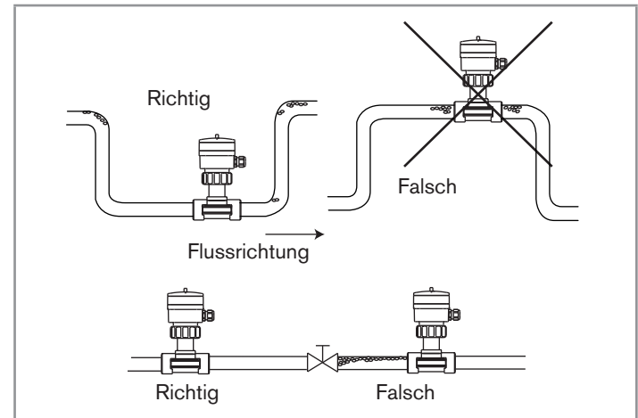
Abb. 7.5 Zusätzliche Installationempfehlungen
