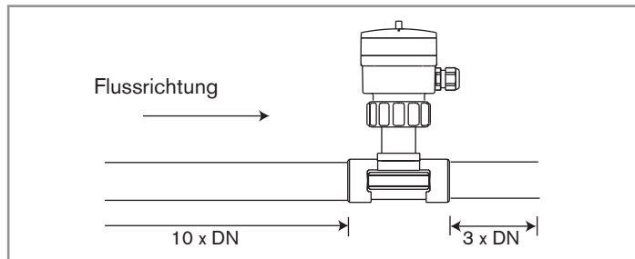
Abb. 7.3: Mindestein- und -auslaufstrecken
