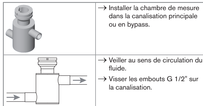
Fig. 7.13 : Installation de la chambre de mesure
