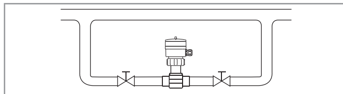
Abb. 7.2: Installation des Fittings im Bypass
