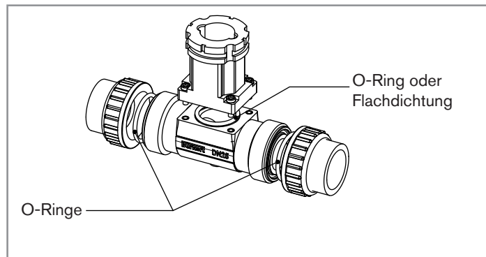
Abb. 11.4: Dichtungen eines T-Fittings mit Klebe- oder Schweißverbindern
