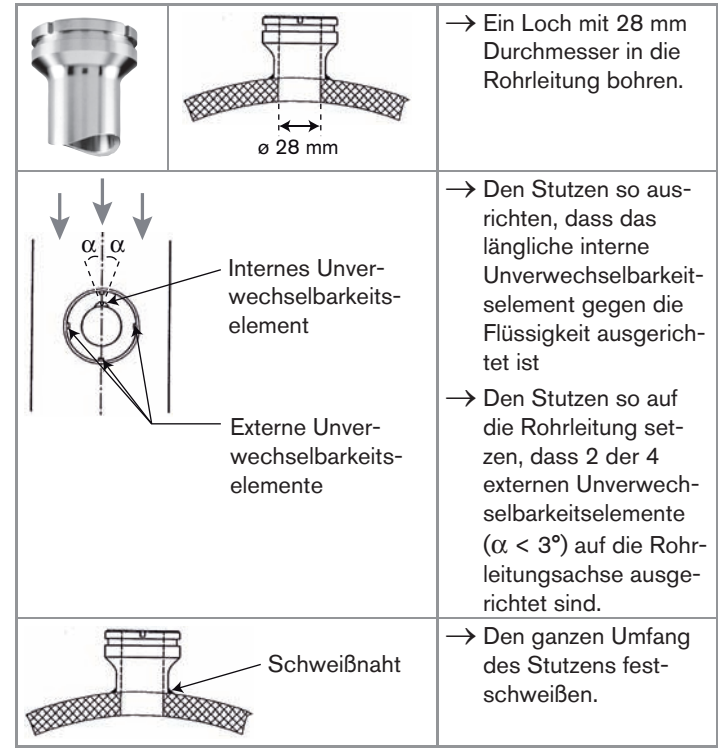
Abb. 7.9: Installation eines Schweißstutzens aus Metall
