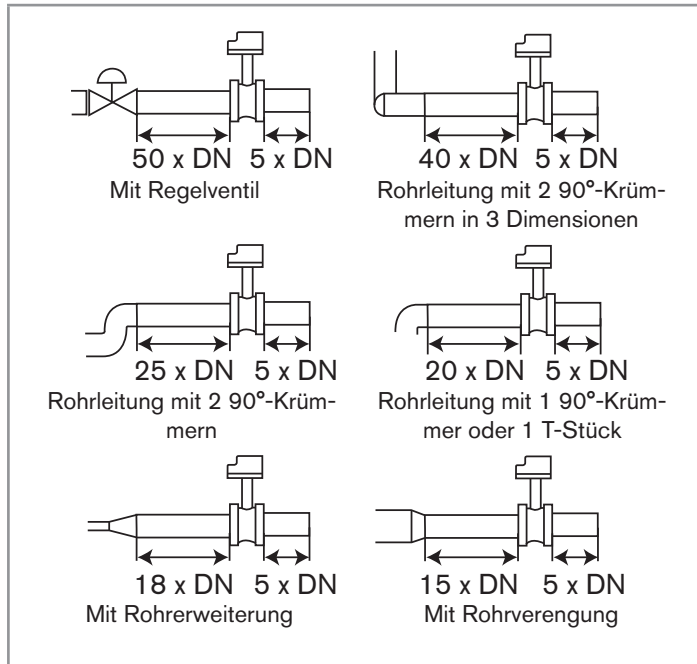
Abb. 7.4: Mindestein- und -auslaufstrecken je nach Aufbau der Rohrleitungen.
