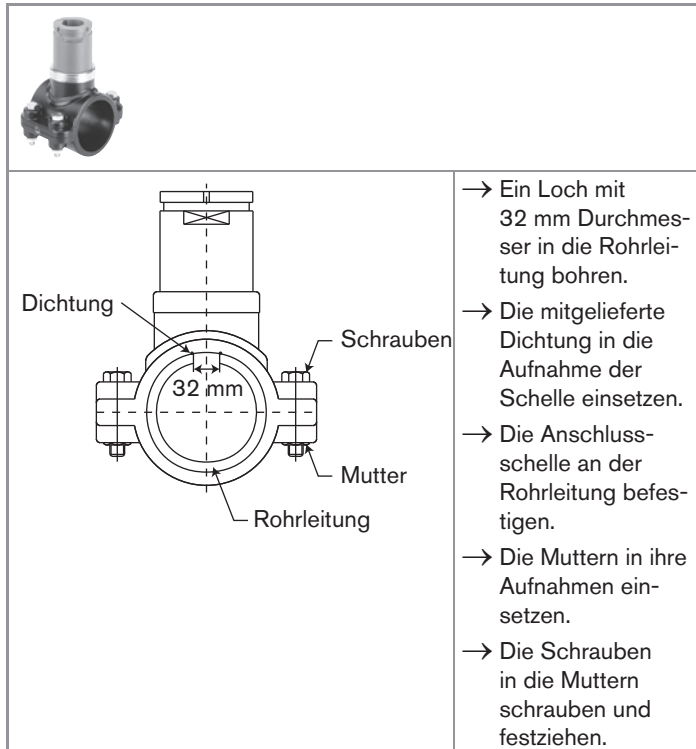
Abb. 7.8: Installation eines Fittings mit Anschlussschellen
