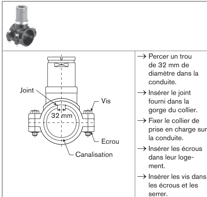
Fig. 7.8 : Installation d'un raccord avec collier de prise en charge
