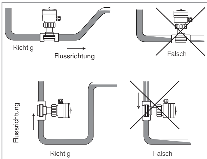
Abb. 7.6 Zusätzliche Installationsempfehlungen
