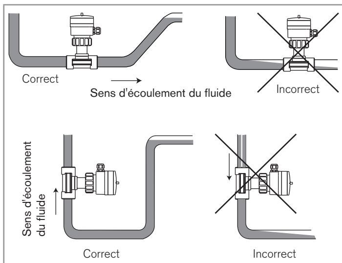
Fig. 7.6 Recommandations additionnelles d'installation
