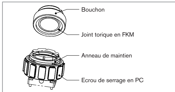
Fig. 11.3 : Bouchon avec joint torique, écrou de serrage et anneau de maintien
