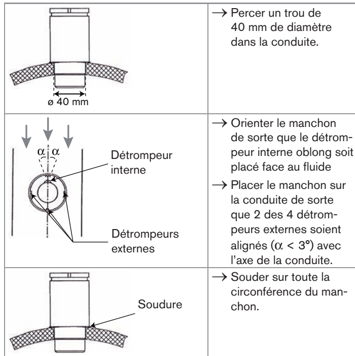
Fig. 7.10 : Installation d'un manchon à souder en matière plastique (PE, PP ou PVDF)
