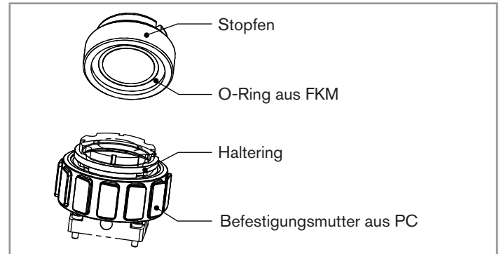
Abb. 11.3: Stopfen mit O-Ring, Befestigungsmutter und Haltering
