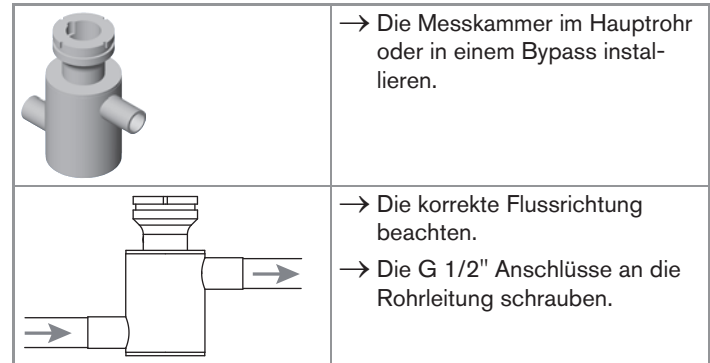
Abb. 7.13: Installation der Messkammer
