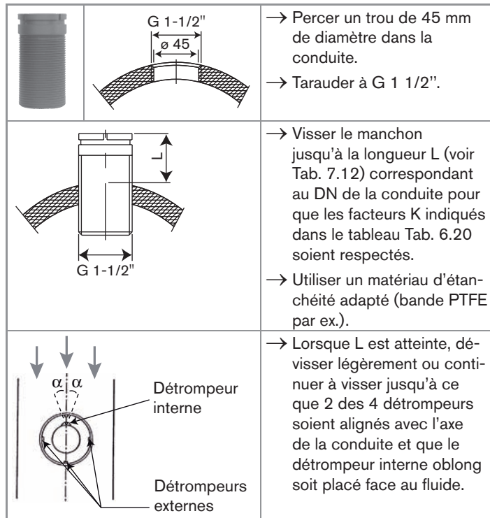
Fig. 7.11 : Installation d'un manchon à visser en matière plastique (PP, PVC, ou PE)
