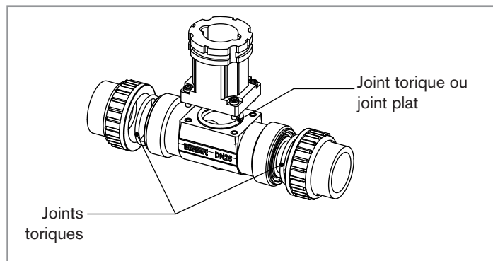
Fig. 11.4 : Joints d'un raccord en T avec embouts union à coller ou à souder
