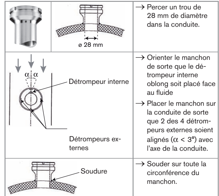
Fig. 7.9 : Installation d'un manchon à souder en métal
