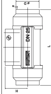
3.4: Acier inox, raccord à souder suivant ISO 4200
